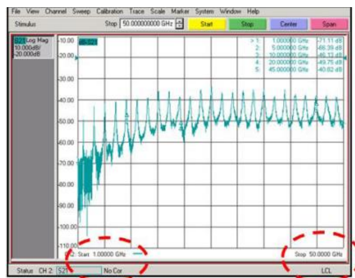
Agilent E8364A PNA 网络分析仪和通用试验夹具 3830 K(由 ANRITSU 提供)用于环形谐振器检测。
